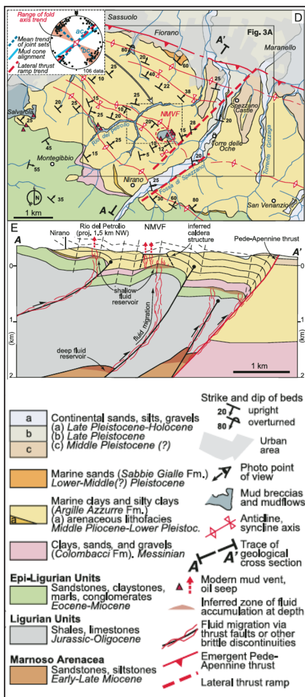
Fig. 6a, 6b - Carta geologico-strutturale e sezione geologica dell'area delle salse di Nirano nel pedeappennino modenese (da BONINI, 2008a) - Geological-structural map and geological cross-section of the Salse di Nirano area in Apennine margin (from BONINI 2008a)
